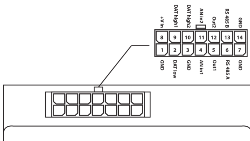
Рис. 3. Расположение разъема и нумерация контактов.
