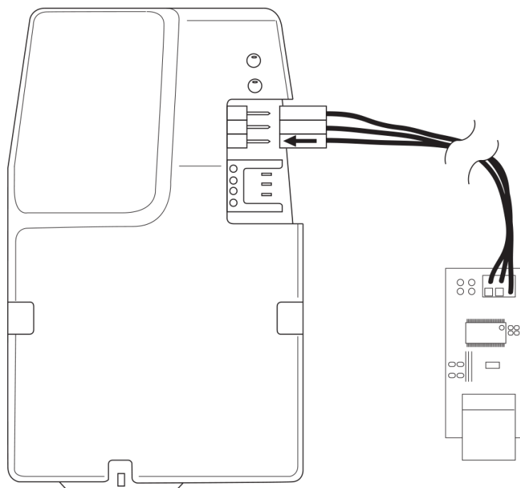
Рис. 4. Подключение кабеля преобразователя USB-UART к устройству BI 520R TREK.
