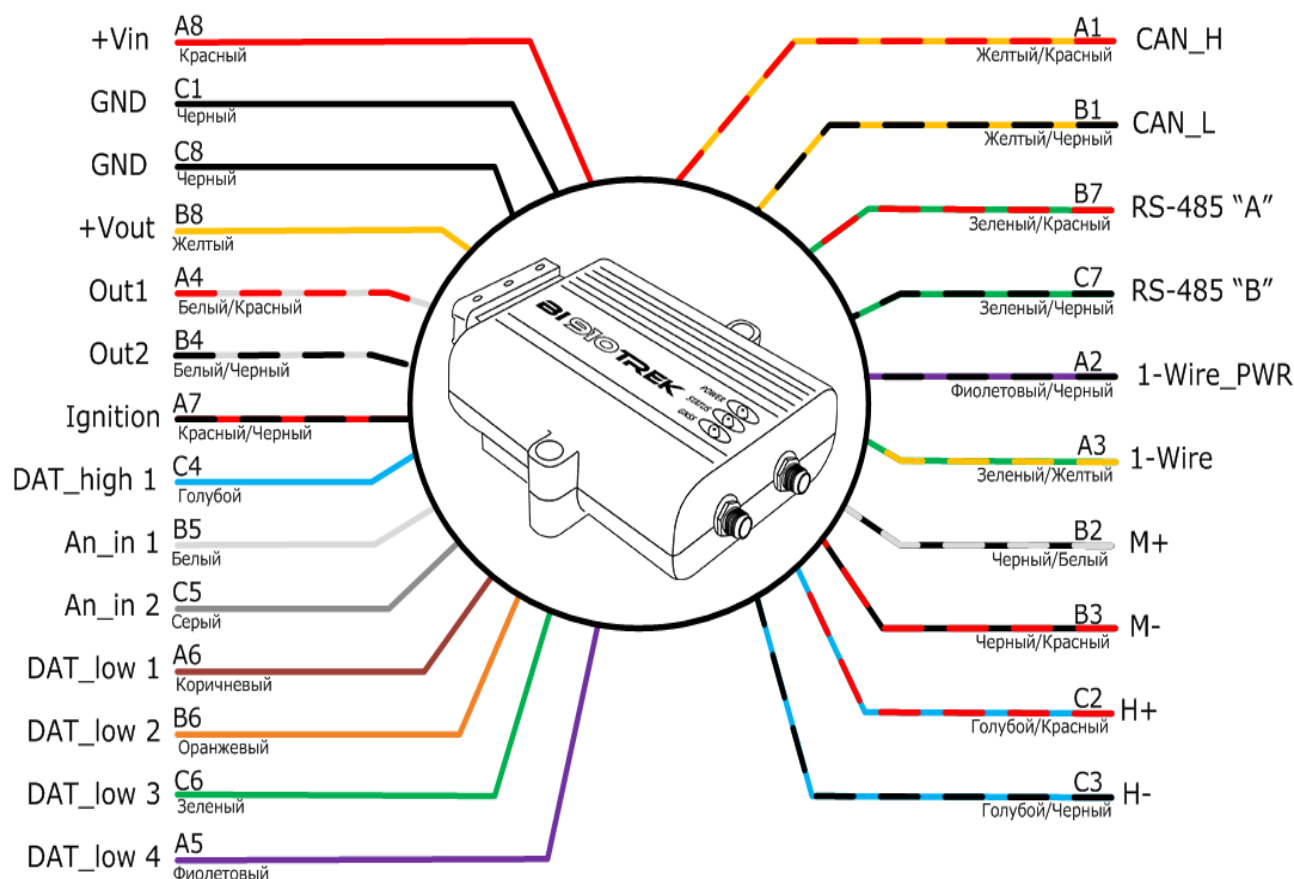
Рис. 5. Назначение контактов BI 910 TREK
