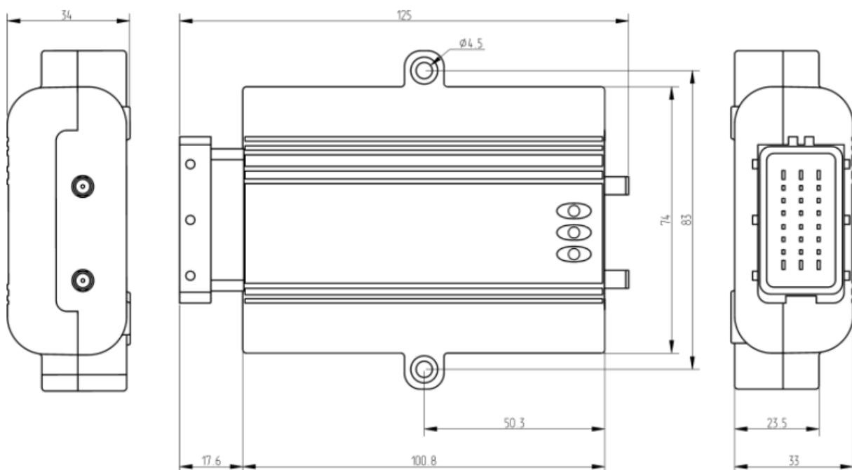
Рис. 1. Внешний вид и габаритные размеры устройства наблюдения «BI 910 TREK». (Общий вид)
