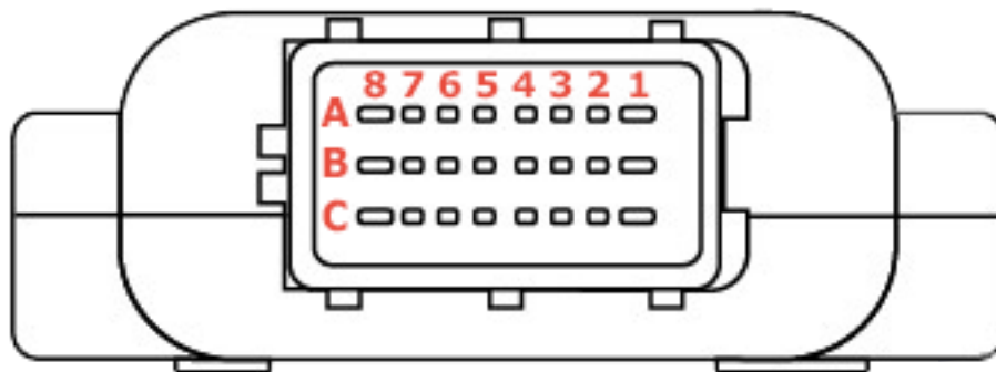
Рис. 4. Расположение разъёма и нумерация контактов
