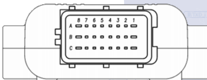
Рис. 2. Внешний вид и габаритные размеры устройства наблюдения «BI 910 TREK». (Вид сзади)
