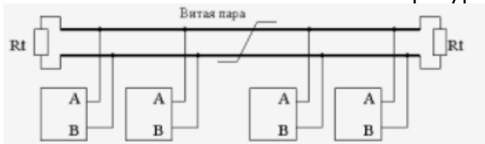
Рис. 10. Схема согласования и конфигурации линии связи А и В.
