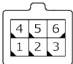
Рис.4. Разъем для подключения внешних устройств
