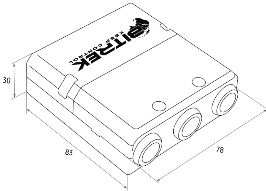
Рис.1. Внешний вид и габаритные размеры
