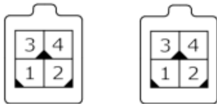
Рис.3. Разъёмы Connect-Bus №1 и №2
